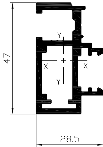
כנף שניה לזיגוג רגיל פרופיל 07328 שטח : 377 ממ"ר משקל : 1018 ג/מ היקף כללי : 319 מ"מ היקף חיצוני : 226 מ"מ I_{xx} = 8.40 \text{ Cm}^4 I_{yy} = 2.36 \text{ Cm}^4
