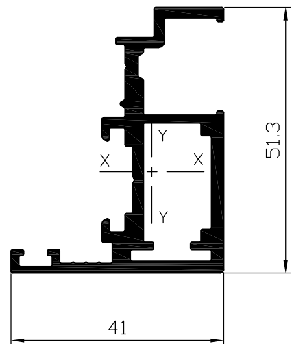
כנף לזיגוג בידודי פרופיל 07323 שטח : 400 ממ"ר משקל : 1080 ג/מ היקף כללי : 355 מ"מ היקף חיצוני : 260 מ"מ I_{xx} = 10.76 \text{ Cm}^4 I_{yy} = 3.66 \text{ Cm}^4
