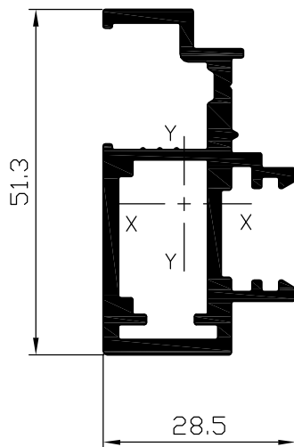
כנף שניה לזיגוג בידודי פרופיל 07329 שטח : 362 ממ"ר משקל : 977 ג/מ היקף כללי : 324 מ"מ היקף חיצוני : 231 מ"מ I_{xx} = 8.77 \text{ Cm}^4 I_{yy} = 2.22 \text{ Cm}^4
