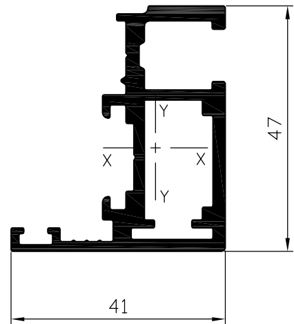
כנף לזיגוג רגיל פרופיל 06991 שטח : 415 ממ"ר משקל : 1121 ג/מ היקף כללי : 350 מ"מ היקף חיצוני : 254 מ"מ I_{xx} = 10.44 \text{ Cm}^4 I_{yy} = 3.86 \text{ Cm}^4
